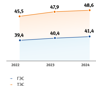
Коэффициент использования установленной мощности ТЭС и ГЭС, %
